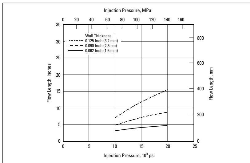
图表 11-10. ULTEM1000 树脂在675° F(357°C)时的 流动长度
