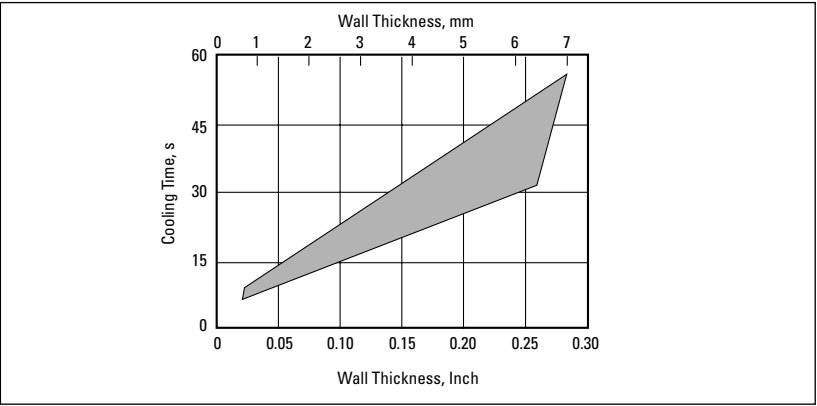
图表 11-9. ULTEM 树脂的冷却时间与壁厚
