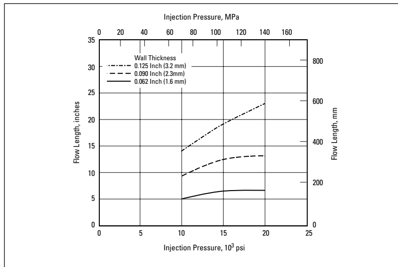
图11-12. 750° F(399℃)时， ULTEM 1000树脂的流动长度
