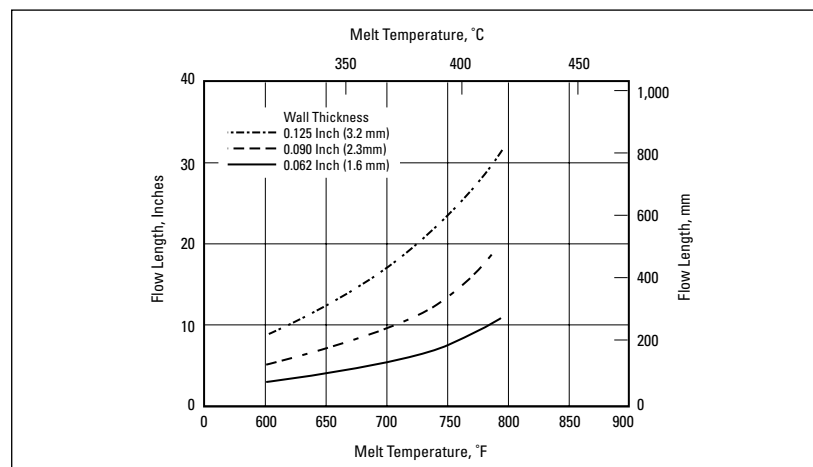
图 11-13. 注射压力为20,000 磅/平方英寸(138兆帕)时， ULTEM 1000树脂的流动长度
