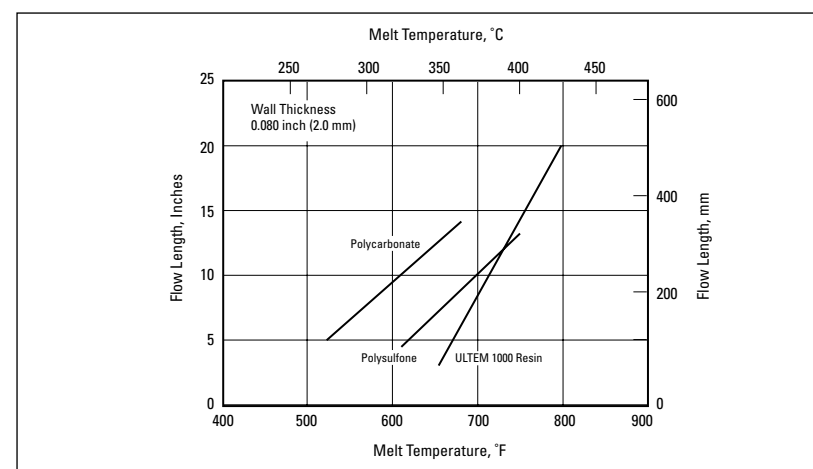
11-14. 熔体温度对ULTEM 1000树脂以及其它热塑性树脂 流动长度的影响。
