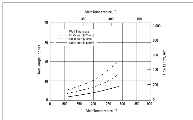
图表 11-11. 注射压力为 10,000磅/平方英寸(69兆 帕)时，ULTEM1000树脂的 流动长度
